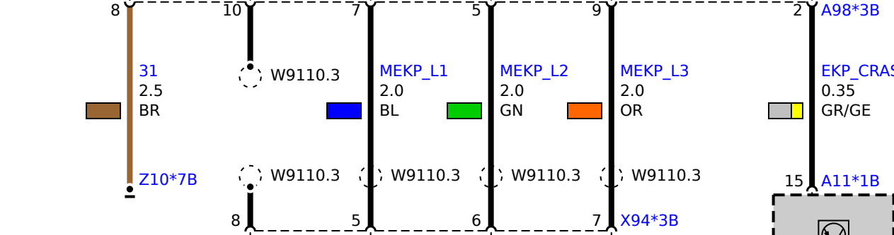
A98*3B EKP_CRAS 0.35 GR/GE A11*1B A11 Crash safety module
