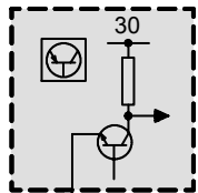
A3 Light module
